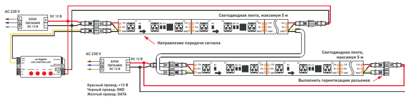
Рис. 1. Схема подключения нескольких светодиодных лент SPI-B60 с двух сторон с использованием SPI-контроллера с одним выходным портом и отдельных блоков питания
