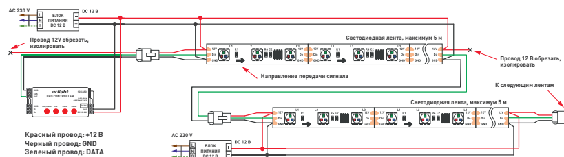
Рис. 4. Схема подключения нескольких светодиодных лент SPI-B60 и SPI-SE-B60 с двух сторон с использованием SPI-контроллера с одним выходным портом и отдельных блоков питания
