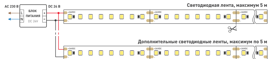
Рис. 1. Подключение нескольких светодиодных лент с одной стороны
