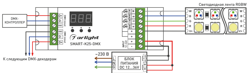
Рис. 1. Общая схема подключения декодера
