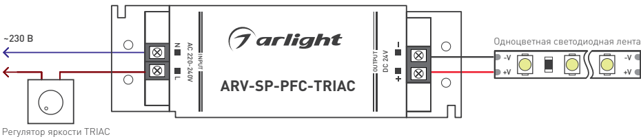
Рис. 1. Пример подключения источника питания
