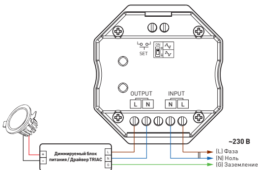
Рис. 4. Схема подключения светодиодных светильников или светодиодной ленты
