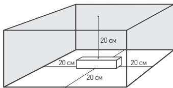
Рис. 1. Свободное пространство вокруг ограничителя
