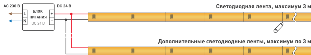
Схема 1. Подключение нескольких светодиодных лент с двух сторон
