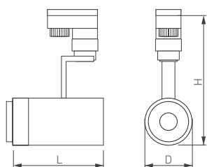
Рисунок 1. Чертеж и габаритные размеры
