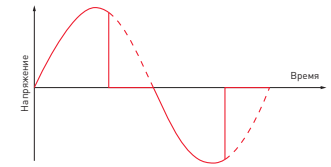
Диммирование с отсечкой заднего фронта. Используется для ламп накаливания и емкостной нагрузки, в том числе светодиодных источников света
