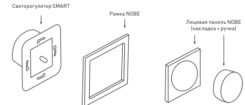
Рис. 5. Монтаж светорегулятора
