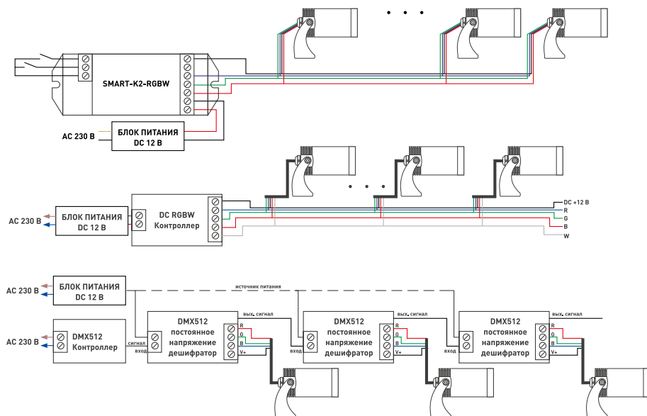
Рис. 2. Схемы подключения
