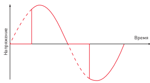
Диммирование с отсечкой переднего фронта. Используется для лам накаливания и индуктивной нагрузки
