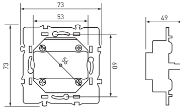
Рис. 1. Габаритный чертеж
