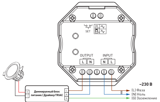
Рис. 4. Схема подключения светодиодных светильников или светодиодной ленты
