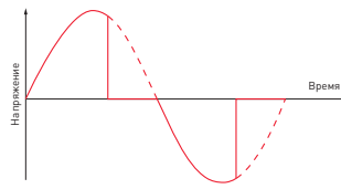
Диммирование с отсечкой заднего фронта. Используется для лам накаливания и емкостной нагрузки, в том числе светодиодных источников света
