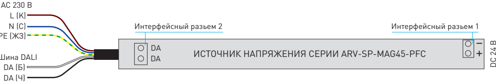
Рис. 1. Схема подключения
