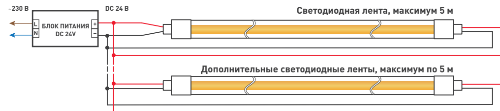
Схема 1. Подключение нескольких светодиодных лент с двух сторон. Рекомендуется использовать для обеспечения равномерного свечения ленты по всей длине
